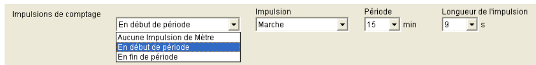
Fig. 87 : Réglages de l'appareil : impulsion de comptage
