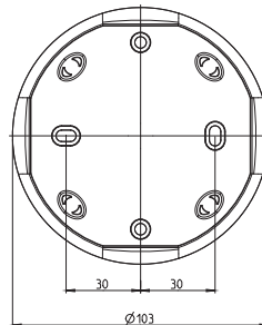
thePrema P360 KNX UP avec boîtier apparent 110A
